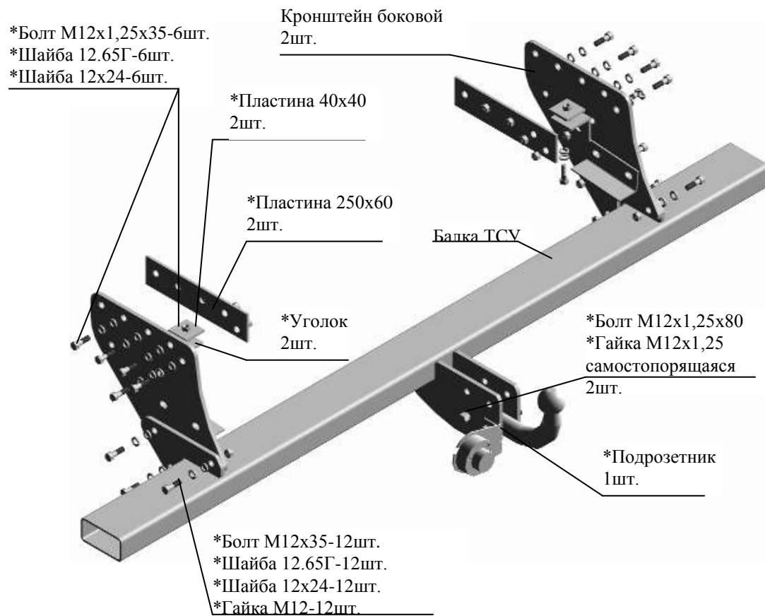
Рис.1 Тягово-сцепное устройство 7110Эж
