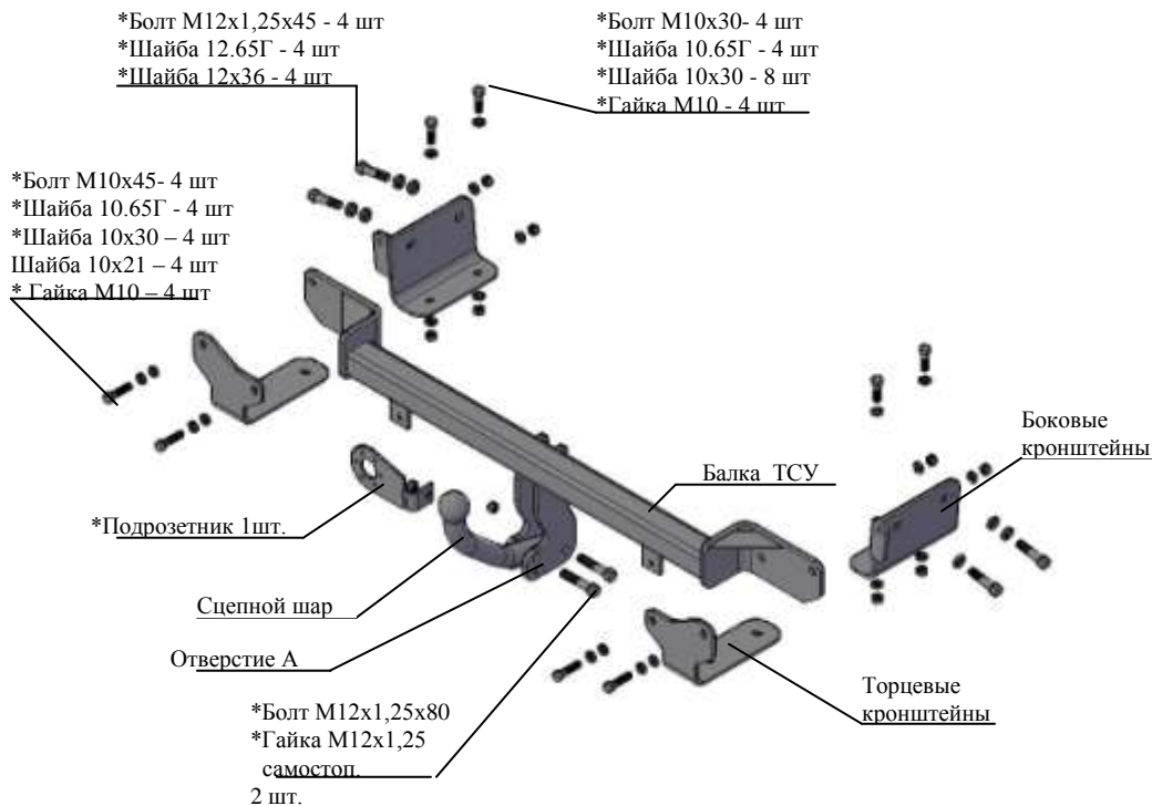
Рис.1 Тягово-сцепное устройство 7330.
