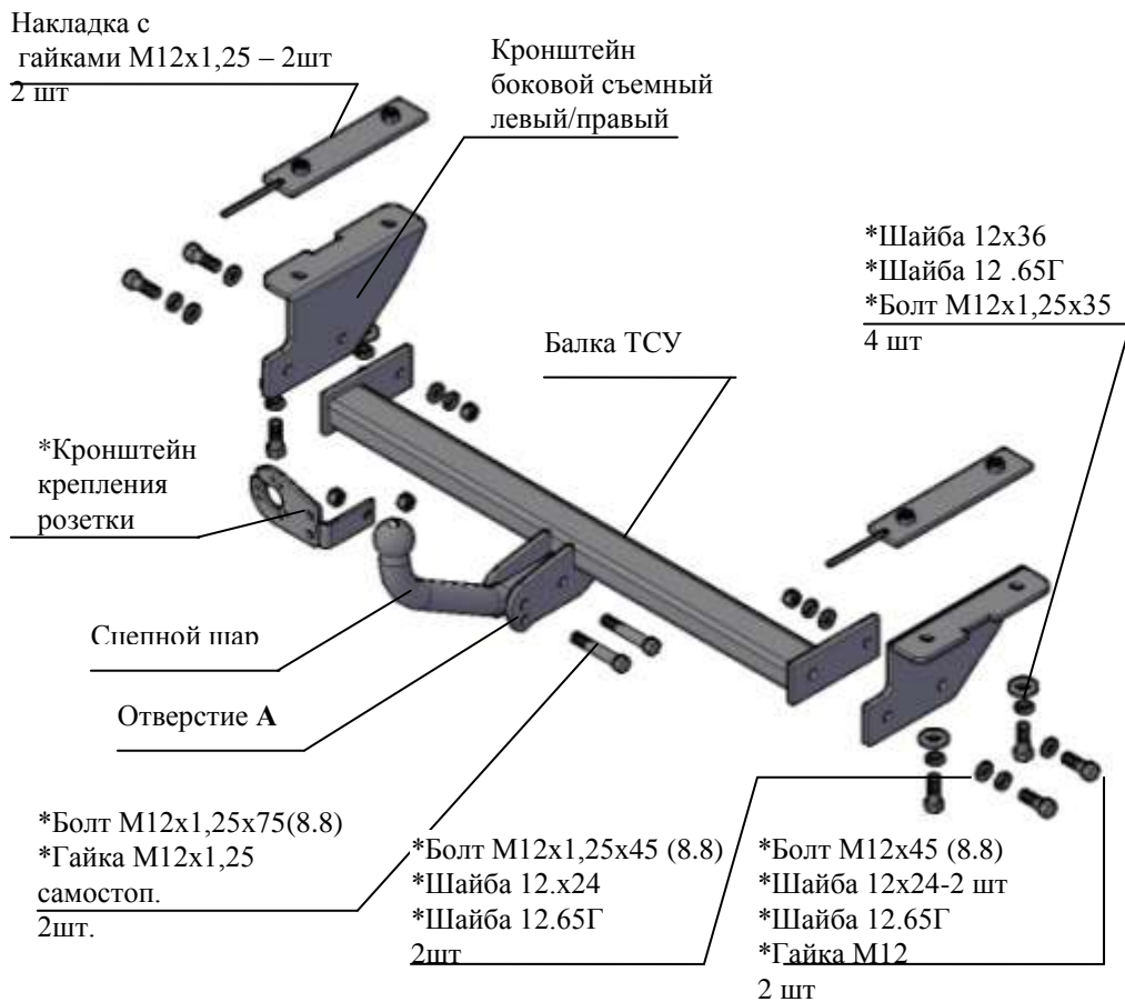
Рис.1 Тягово-цепное устройство 8220
