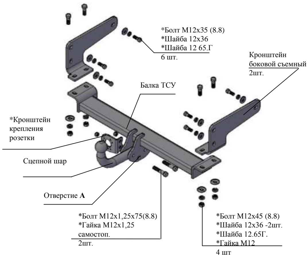
Рис.1 Тягово-сцепное устройство 9910
